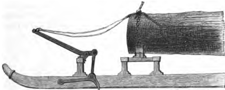
Fig. 191.—Wasenmeister's brake.
